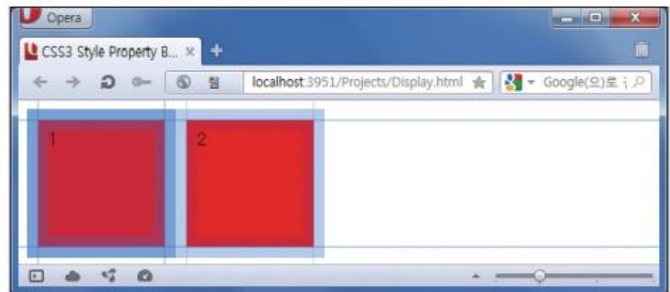
그림 4-90 float 속성에 left 키워드 적용
